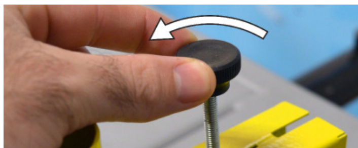
Fig.75 - Levantando o protetor de serra
