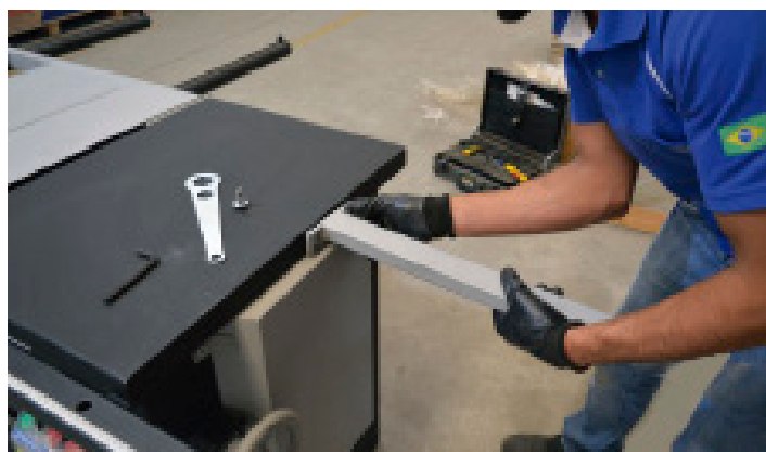
Fig.20 - Colocando o prolongador
