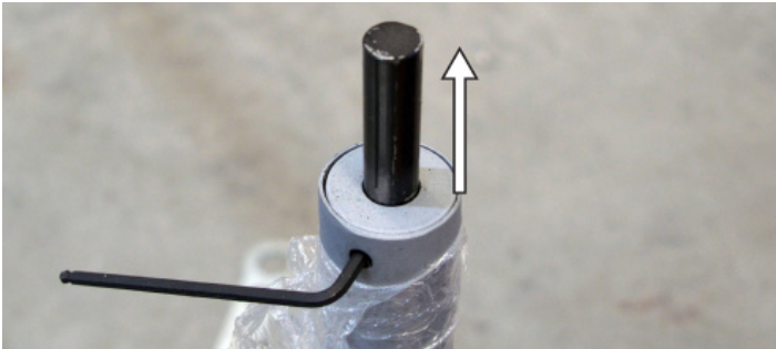
Fig.6 - Afrouxando o parafuso e levantando os pinos dos pés.
