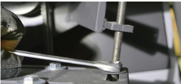
Fig.85 - Esticando as correias apertando a porca da haste na base do motor
