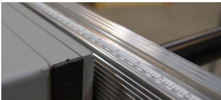
Fig.78 - Detalhe da guia rebaixada
