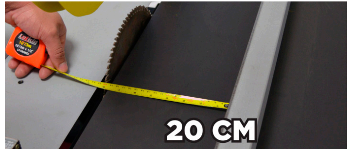
Fig.87 - Medindo a entrada da serra
