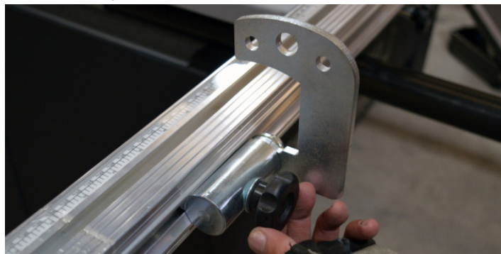
Fig.82 - Manípulo do sistema stop
