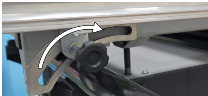
Fig.80 - Desligando a guia para a direita
