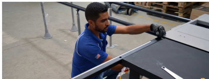
Fig.17 - Prendendo a guia fixa
