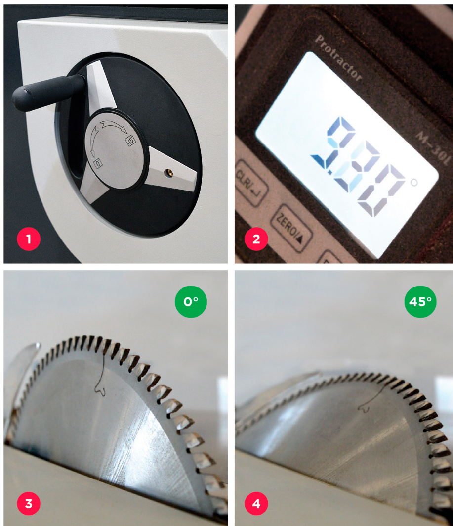
Fig. 1: Volante de inclinação: Gire-o no sentido horário para inclinar a serra.
