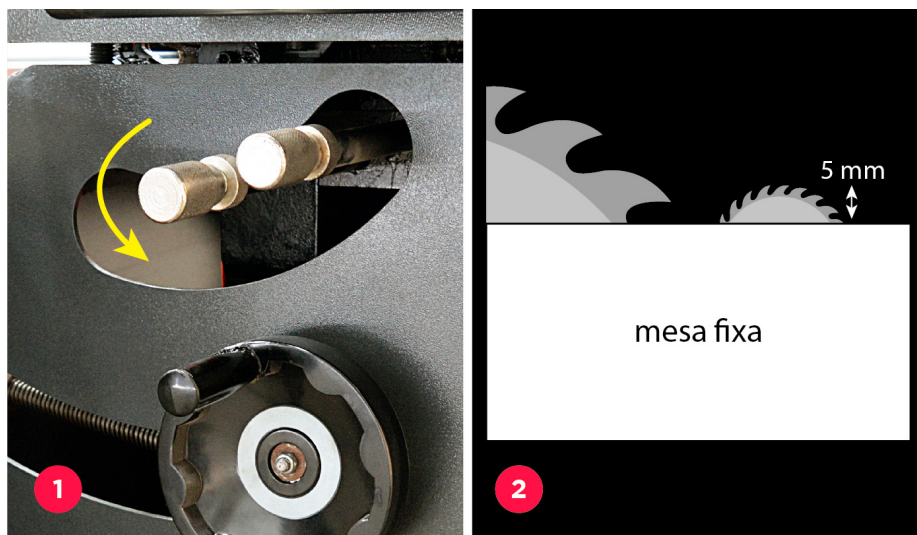
Fig. 1: Manípulo que levanta o riscador.
