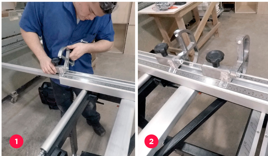
Fig. 1 e 2: Encaixe o sistema stop na guia em alumínio e aperte os manípulos.
