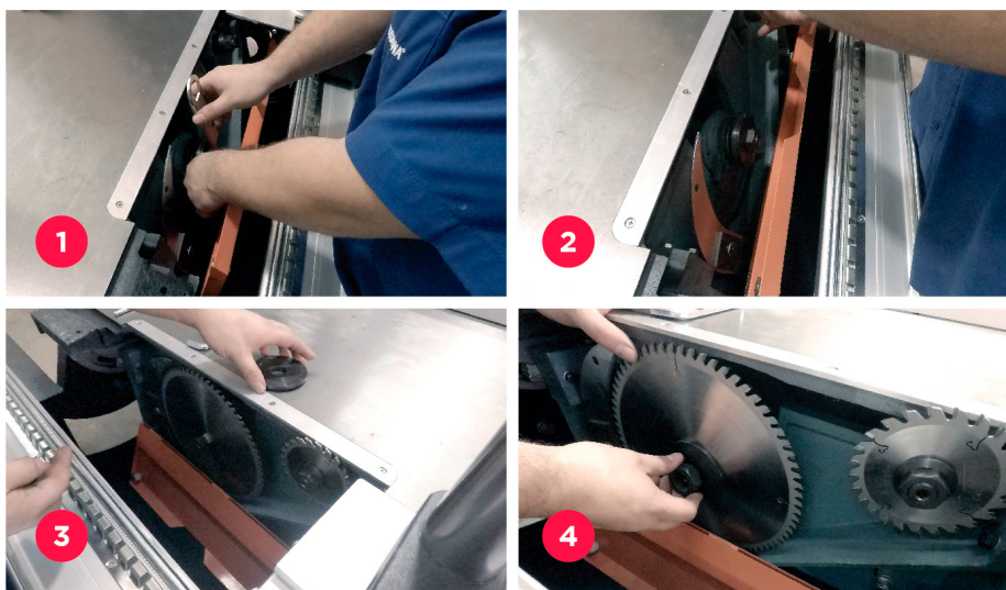
Fig. 1 e 2: Retire a porca e a roldana do sistema de corte.
